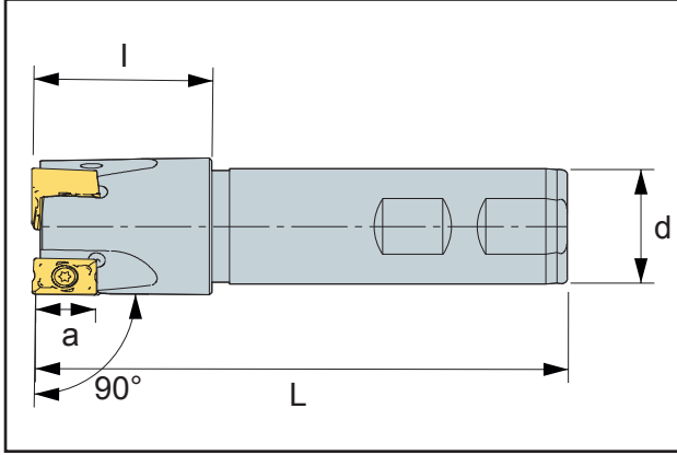
LNMX10 KORLOY / KLP
