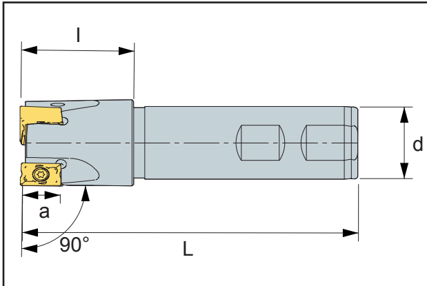
LNMX15 KORLOY / KLP
