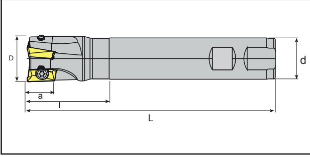
AP.. 11T3.. KORLOY-ZCC
